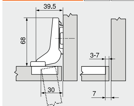
Ușă încadrată
