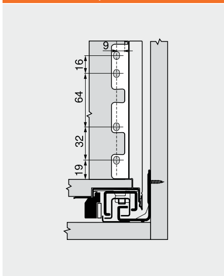
Cote de montare - spate sertar
