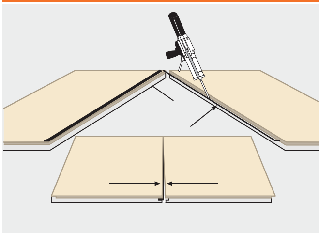
Aplicarea adezivului
