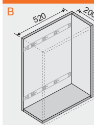
Dimensiuni minime corp
