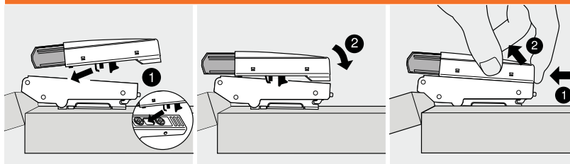
Montare
