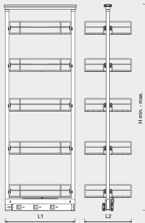
Detalii tehnice
