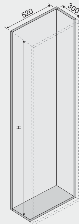
Dimensiuni minime corp
