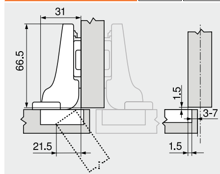
Ușă semiaplicată
