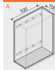
Dimensiuni minime corp
