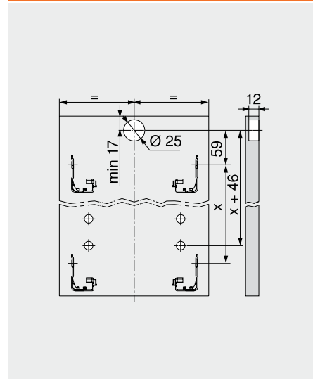
Cote de găurire - front - piesă de antrenare
