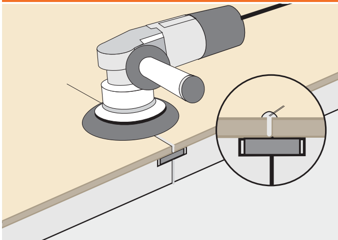
Finisarea suprafeței
