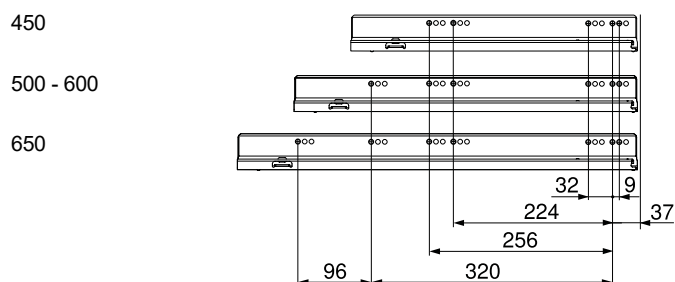
Cote fixare - șină de corp 753 – 70 Kg
