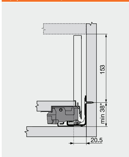
Spațiu necesar în corp
