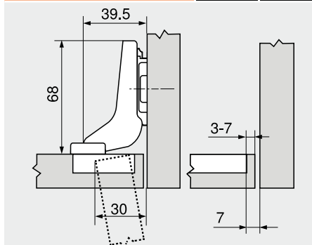
Balama CLIP top BLUMOTION 110° în varianta negru onix.
