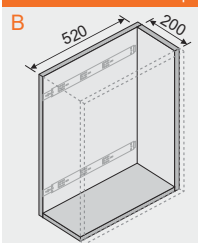
Dimensiuni minime corp
