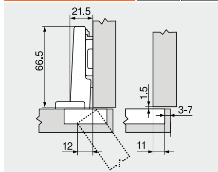
Ușă aplicată
