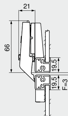
Balama intermediară CLIP top pentru ramă de aluminiu
