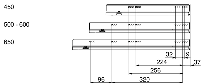
Cote fixare - șină de corp 753 – 70 Kg
