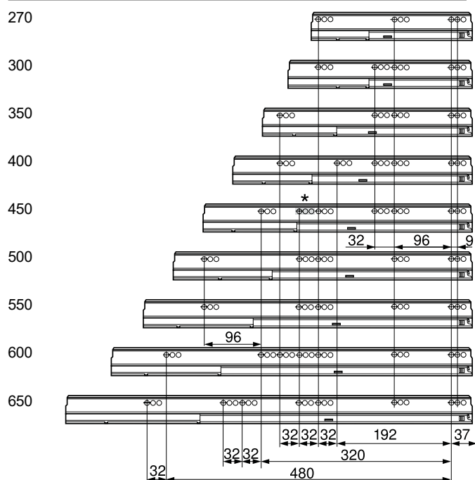
TANDEMBOX antaro sertar interior extragere totală - K
