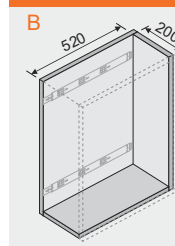
Dimensiuni minime corp
