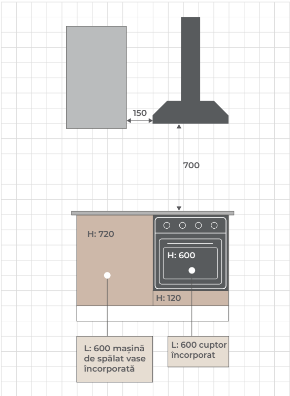
Indicații așezare cuptor:
