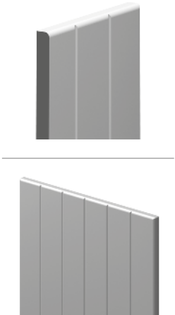
SECȚIUNE - R6: Prelucrare pe contur cu raza 6 mm. Dimensiunile sunt calculate în mm.
