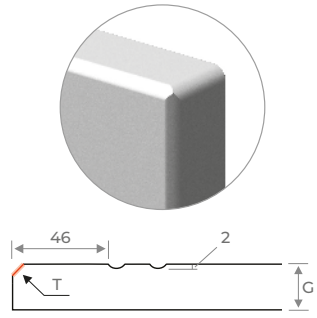
SECȚIUNE - T: Prelucrare pe contur teșit. Dimensiunile sunt calculate în mm.
