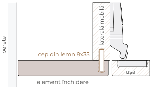
Montare element de închidere vertical
