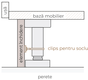
Montare element de închidere vertical
