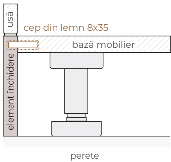
Montare element de închidere vertical
