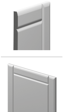
SECȚIUNE - S: Prelucrare pe contur săpun. Dimensiunile sunt calculate în mm.
