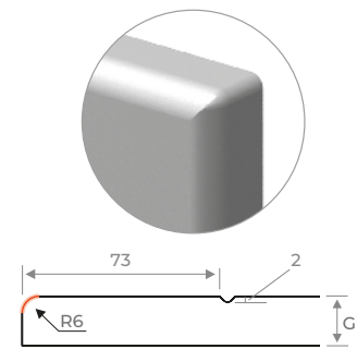
SECȚIUNE - R6: Prelucrare pe contur cu raza 6 mm. Dimensiunile sunt calculate în mm.
