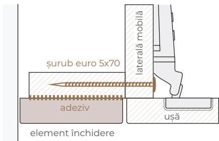
Montare element de închidere vertical
