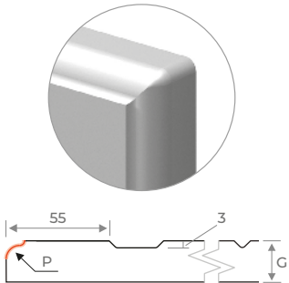
SECȚIUNE - P: Prelucrare pe contur plătuit. Dimensiunile sunt calculate în mm.
