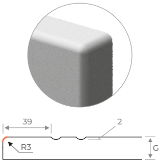
SECȚIUNE - R3: Prelucrare pe contur cu raza 3 mm. Dimensiunile sunt calculate în mm.
