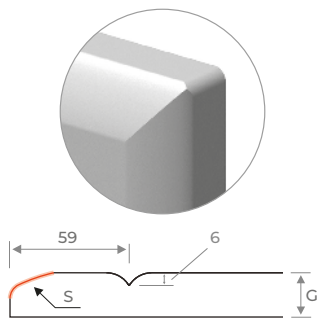
SECȚIUNE - S: Prelucrare pe contur săpun. Dimensiunile sunt calculate în mm.
