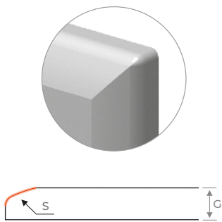
SECȚIUNE - S: Prelucrare pe contur săpun.
